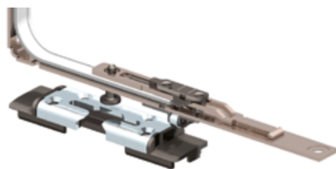
Releveur d'ouvrant progressif et silencieux avec double roulette intégrée
