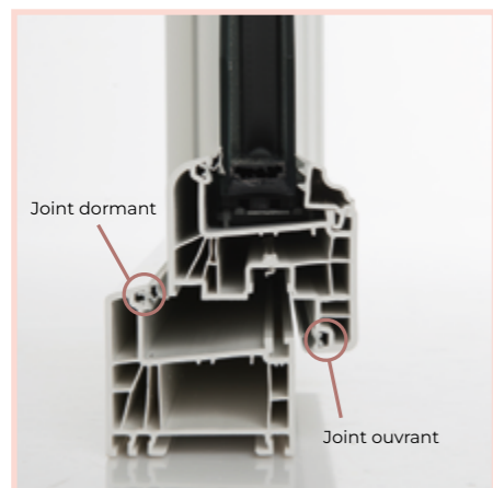
2 JOINTS D'ISOLATION
