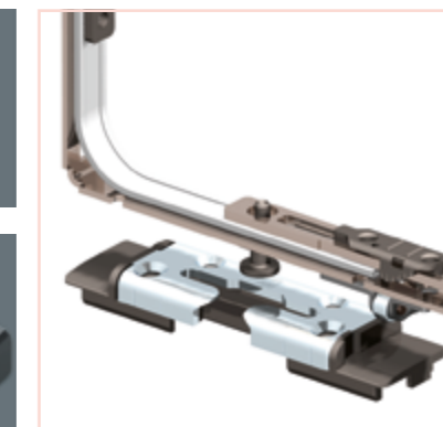
Releveur d'ouvrant progressif et silencieux avec double roulette intégrée
